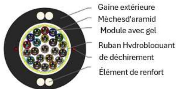
* Schéma de construction typique - pas à l'échelle
